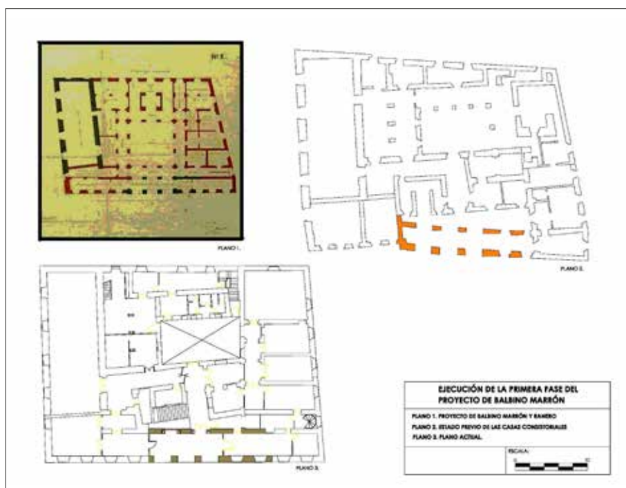
Fig. 4. Ejecución de la primera fase del Proyecto de Balbino Marrón. 1863. Plano: Manuel Buzón Alarcón.
