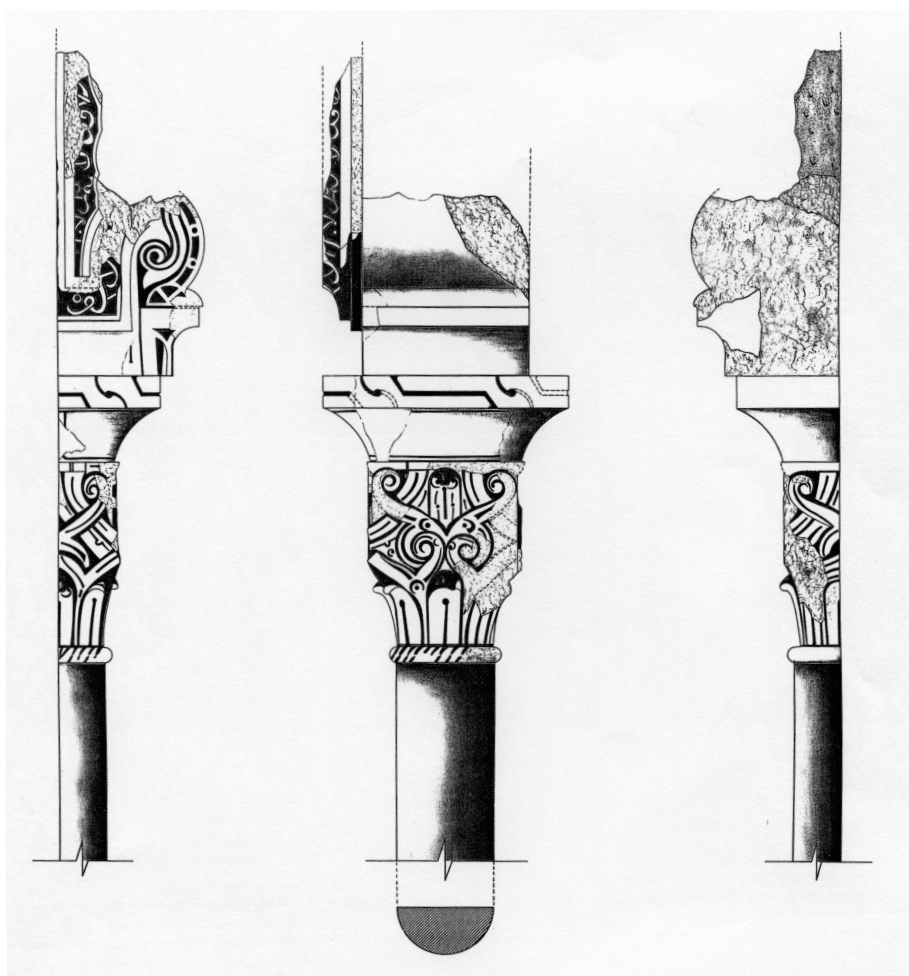
FIG. 10. Murcia. Convento de santa Clara. Alcázar Sagir. Capitel (J. Navarro Palazón).
