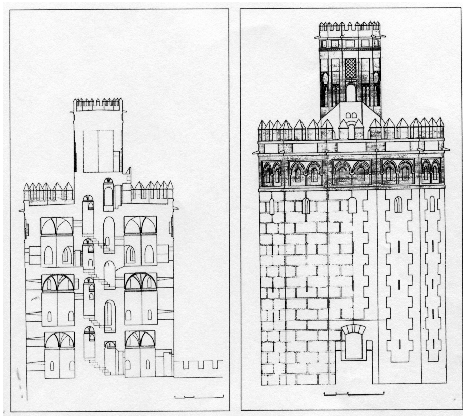
FIG. 17. Sevilla. Torre del Oro. Sección y alzado (B. Pavón Maldonado).
