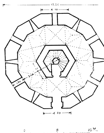
FIG. 7. Sevilla. Torre del Oro. Planta (L. Torres Balbás).
