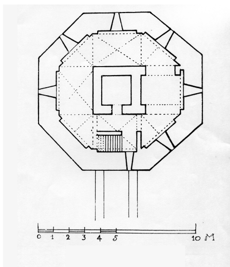
FIG. 6. Badajoz. Torre de Espantaperros. Planta (L. Torres Balbás).
