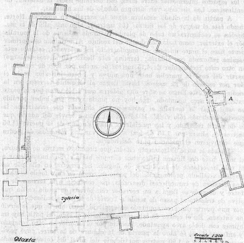
Dib. 6.º—Planta del castillo de Fregenal de la Sierra (Badajoz).
