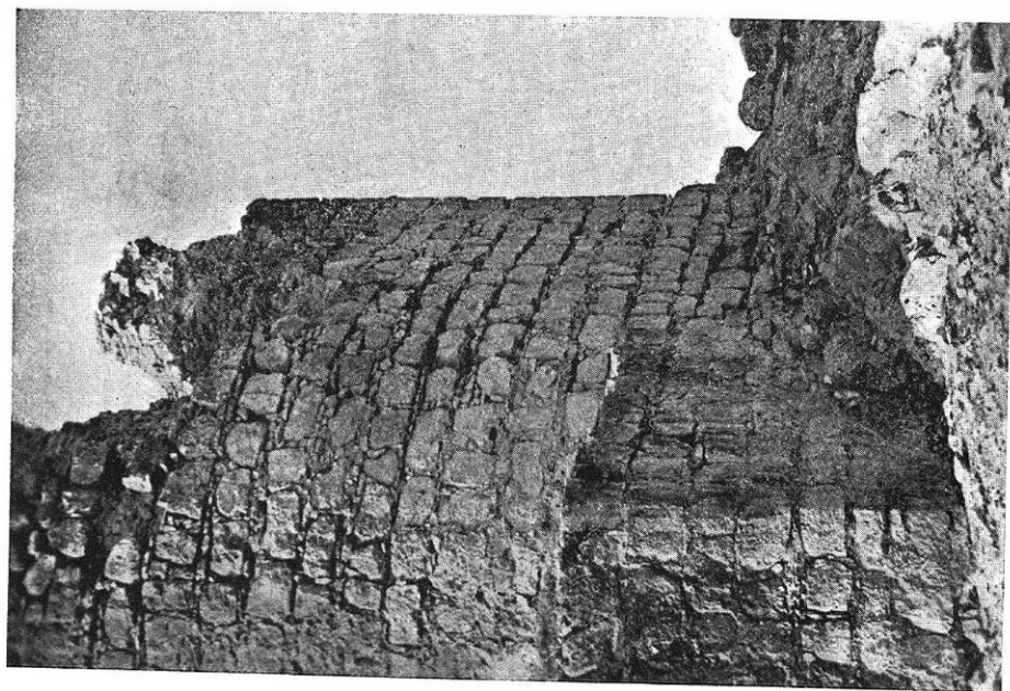
Lám. 11. —Castillo de Cote (Montellano, Sevilla), visto por el ángulo NE. del torreón. (Págs. 126 y 133).
