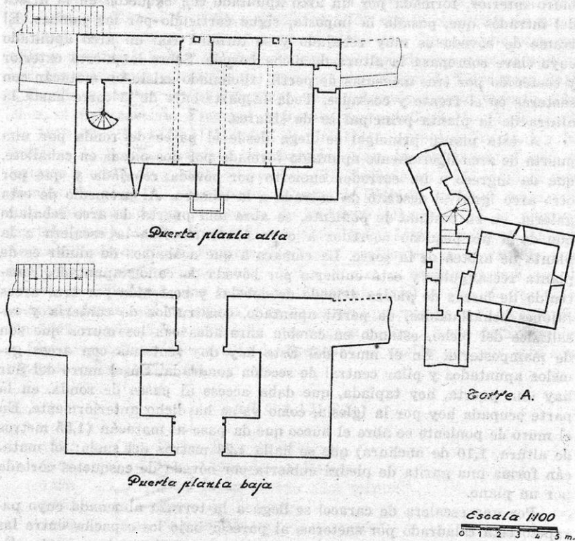
Dib. 7.º.—Plantas de la puerta y torre NE. del castillo de Fregenal de la Sierra (Badajoz).
