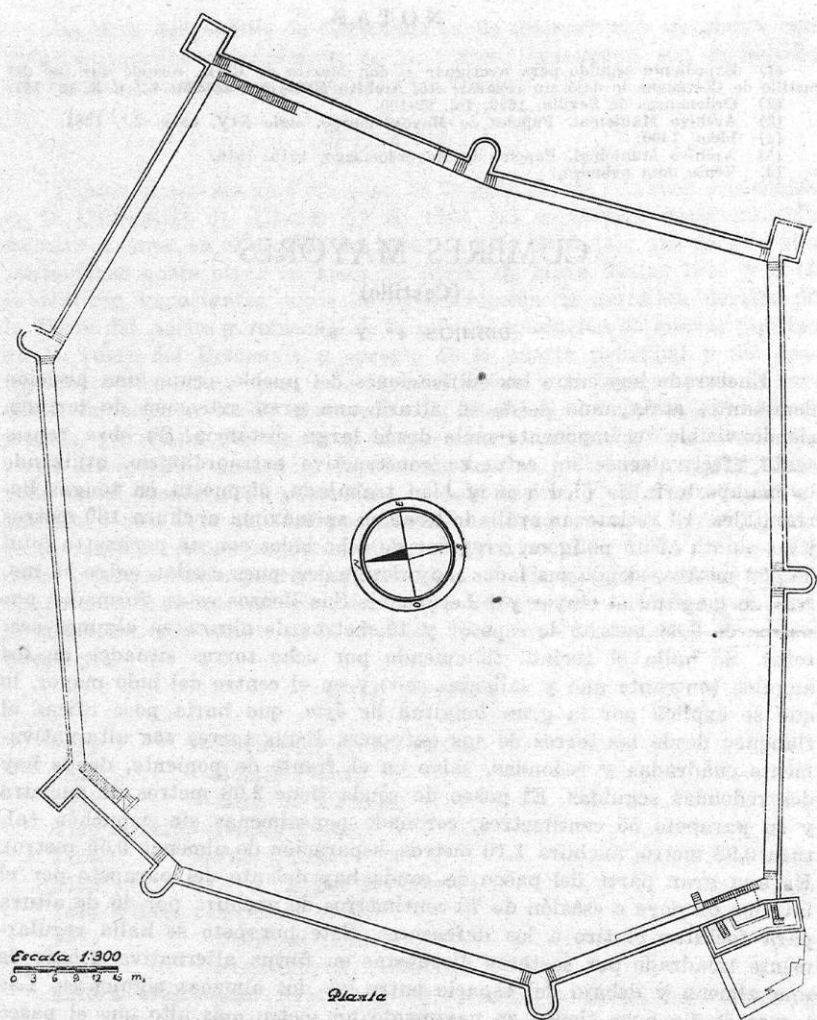
Dib. 4.º—Planta del castillo de Cumbres Mayores (Huelva).
