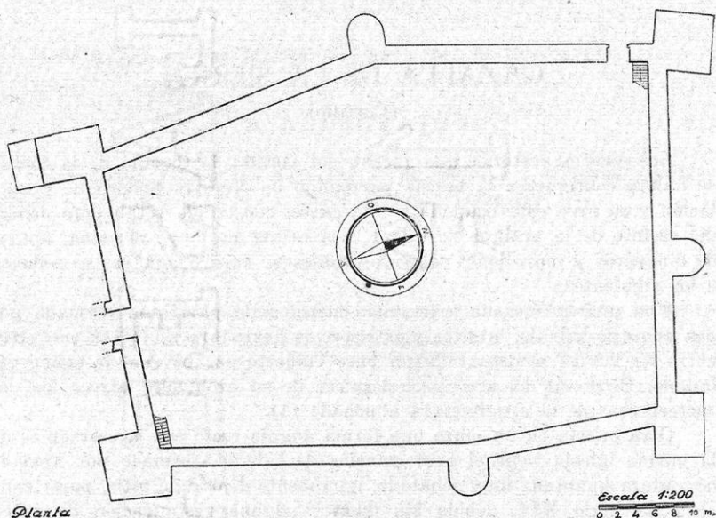
Dib. 2.º —Planta del castillo de Cala (Huelva).
