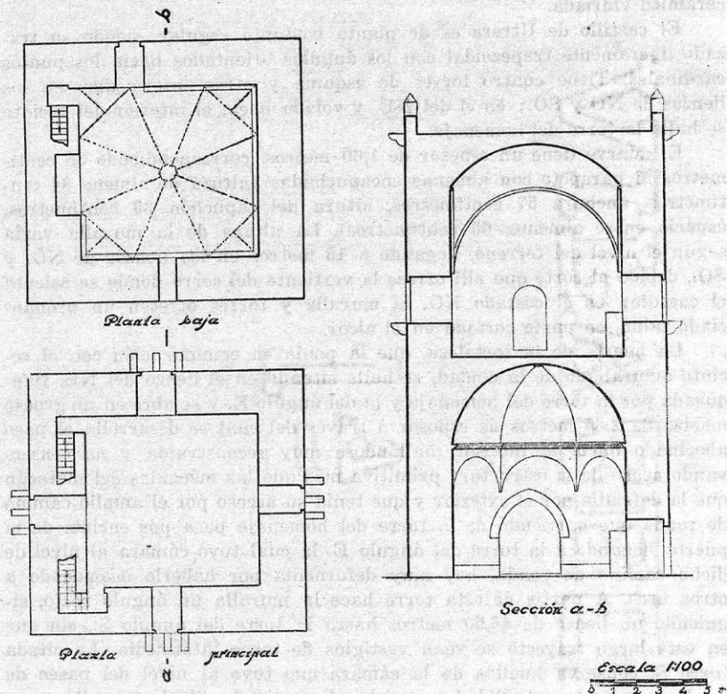
Dib. 13.—Plantas y sección de la torre del homenaje del castillo de Utrera (Sevilla).
