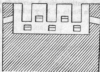
Torre del ángulo S.O. Sección
