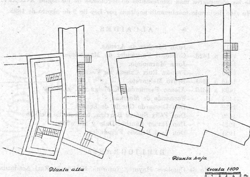
Dib. 5.º—Plantas de la puerta principal del castillo de Cumbres Mayores.
